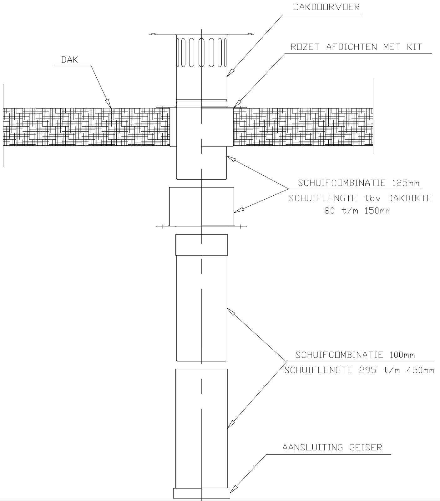
SAMENSTELLING DAKDOORVOER
